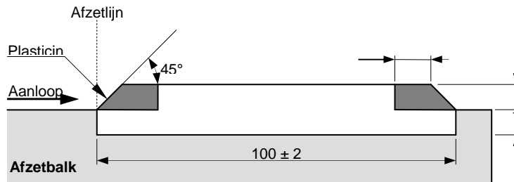
Fig. 10b Plasticinehouder (IAAF) (alle afmetingen in mm)
